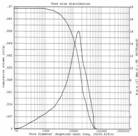
シャモット 55.6%調合焼成素地の細孔分布
