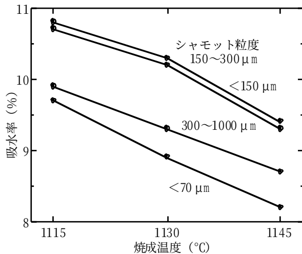
図4 シャモット粒度と吸水率との関係
