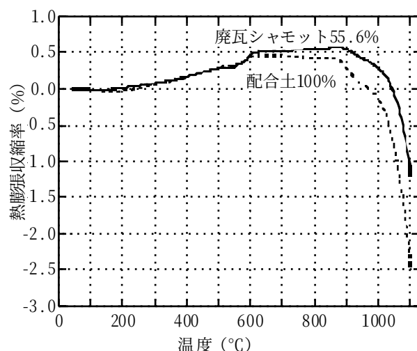
図3 廃瓦シャモット調査素地の熱膨張収縮曲線
