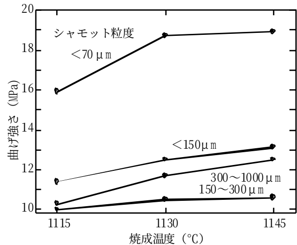
図6 シャモット粒度と曲げ強さとの関係
