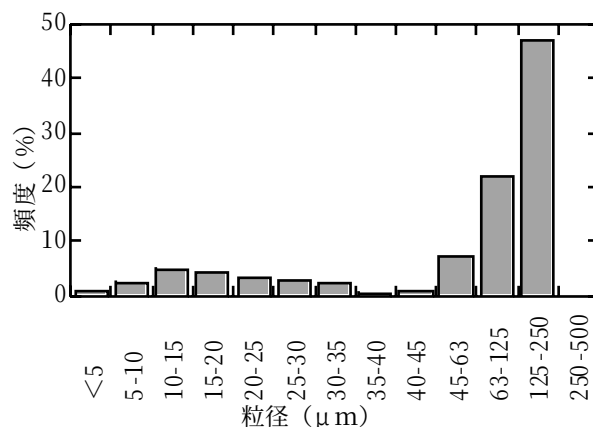
図1 いぶし廃瓦シャモット(150μm以下)粒度
