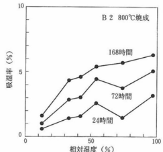
図5 板戸ゼオライト系の吸湿率
