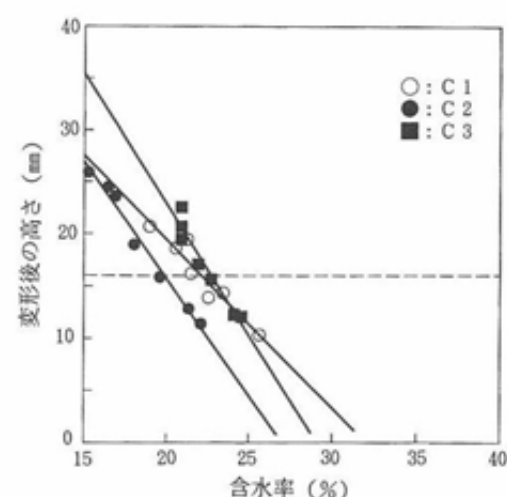
図3 下水道汚泥溶融スラグのベッファーコルンの成形水分
