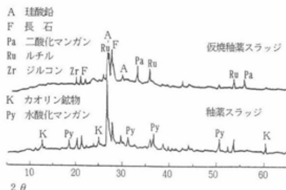
図5 釉薬スラッジのX線回折図(CuK \alpha )
