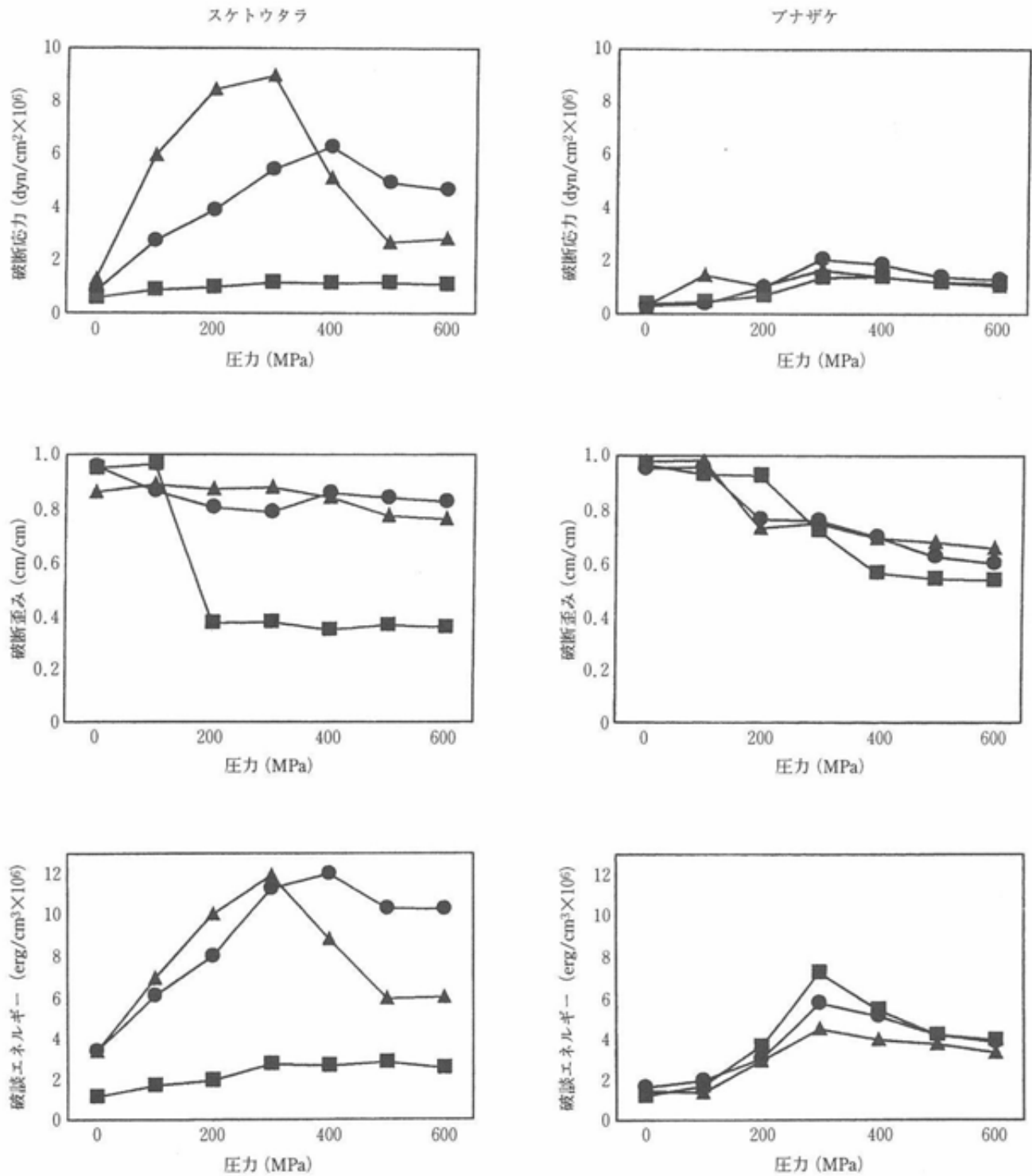
図2 高圧処理後の物性
