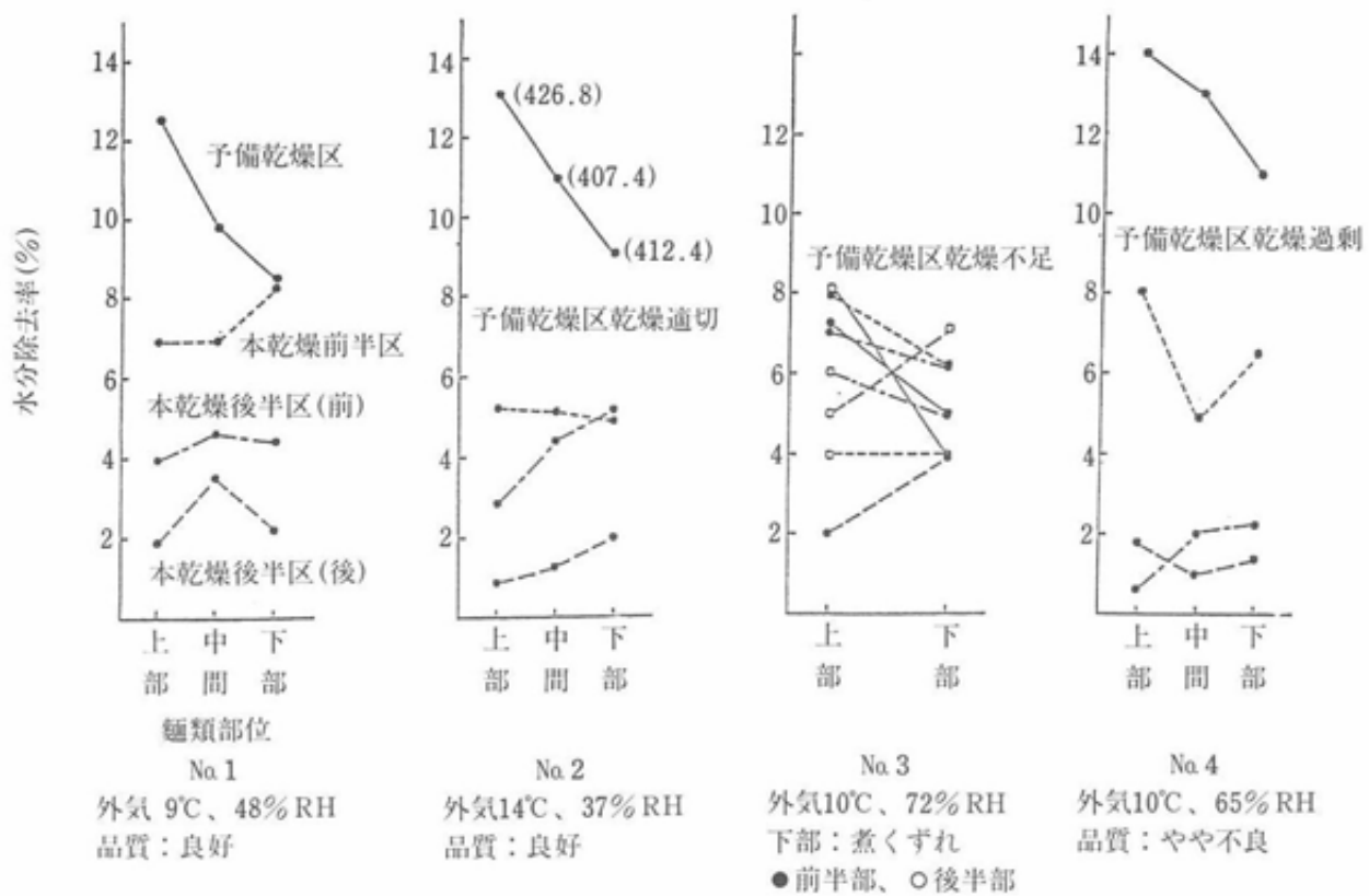
第8図 各乾燥区画における水分除去率(常法)と品質との関係。
