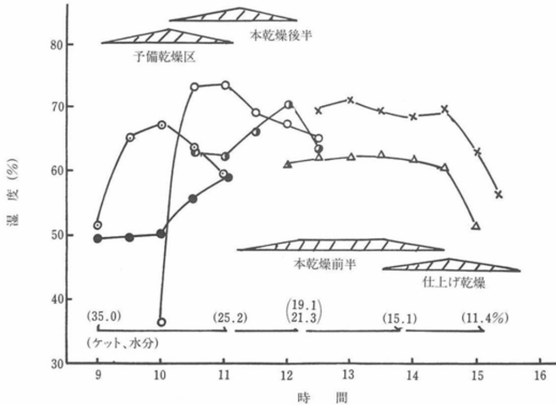
第5図 各乾燥区画の湿度の経時変化
