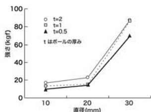
図2 セラミック中空ボールの圧縮強度
