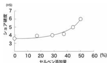
図3 セルベン添加量とショア硬度
