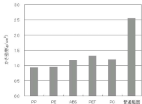
図3 プラスチック樹脂のかさ密度
