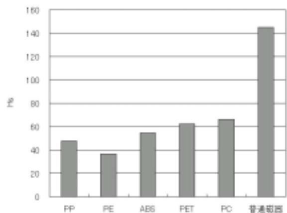
図4 プラスチック樹脂のショア硬さ
