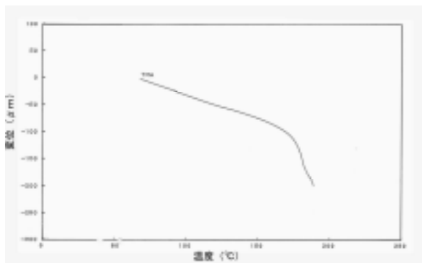
図5 PP樹脂の線膨張変化
