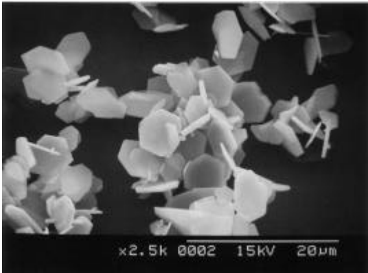
写真4 板状アルミナ (合成物)
