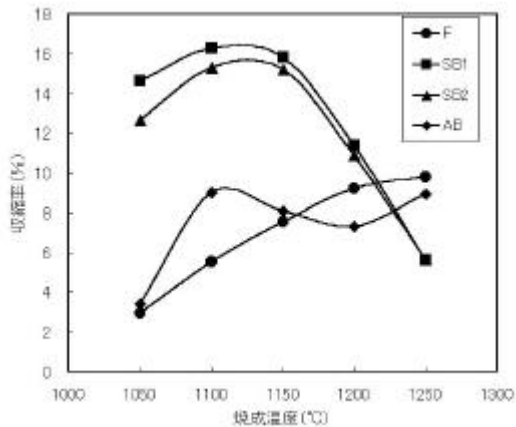
図2 焼成収縮率
