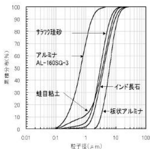
図1 使用原料の粒度分布
