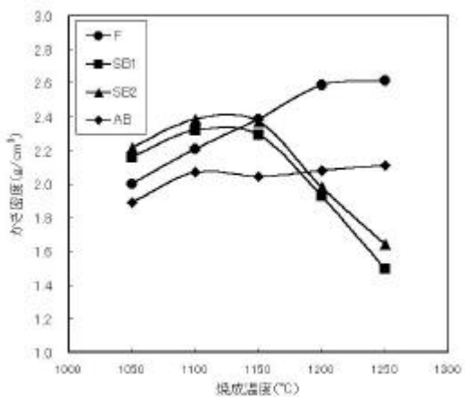
図3 かさ密度
