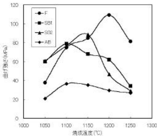
図4 曲げ強さ
