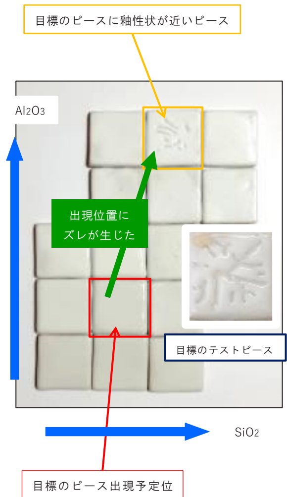
図3 梅花皮釉の再現試験 (9点調査試験)
