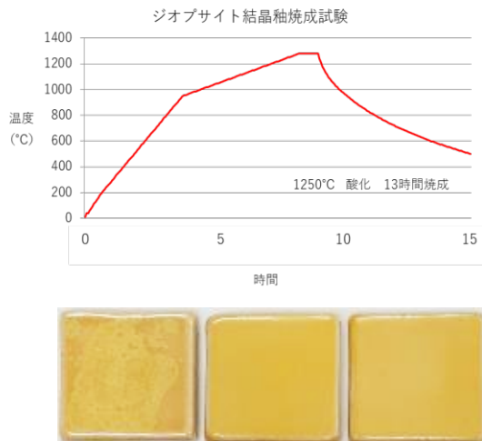
図4 1250°C焼成、自然冷却の焼成グラフと焼成したテストピース
