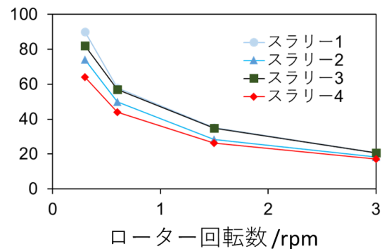
図 3 B 型粘度計を用いた粘度測定 (含水比を 30%に揃えて測定)
