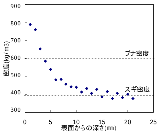
図1 密度分布（30%圧縮スギ材）
