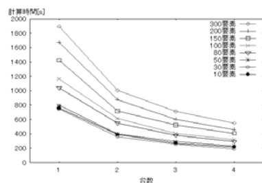
図4 計算台数と計算時間の関係
