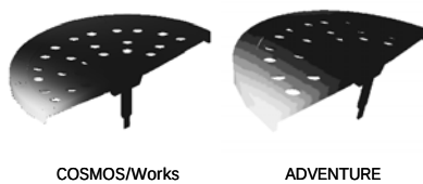
図7 割り出しテーブルにおける合成変位量
