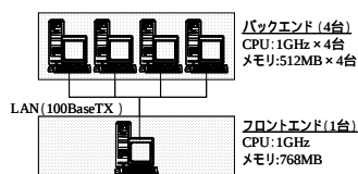
図1 システム構成
