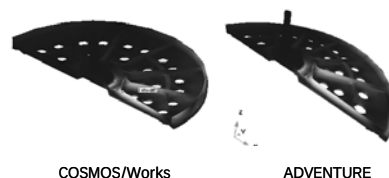
図6 割り出しテーブルにおける応力分布図
