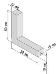
図2 L字型梁モデル
