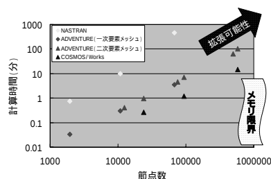
図5 節点数と計算時間の関係
