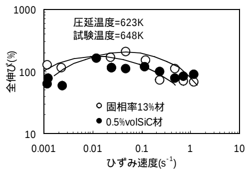
図8 ひずみ速度と全伸びの関係
