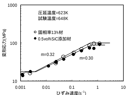
図7 ひずみ応力と変形応力の関係
