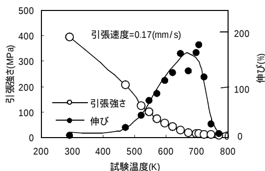
図6 試験温度と引張強さ、伸びの関係
