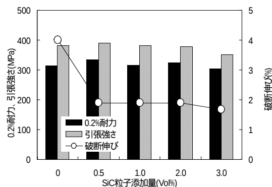
図3 SiC粒子添加量と引張強さ、0.2%耐力及び伸びの関係
