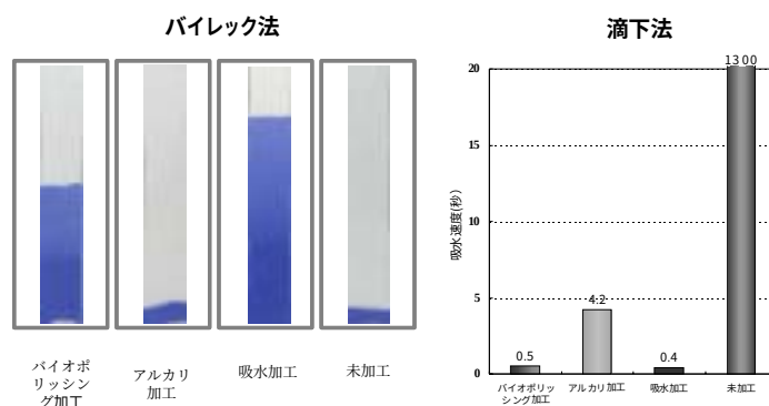
図4 各種加工処理を施したPET布の吸水性
