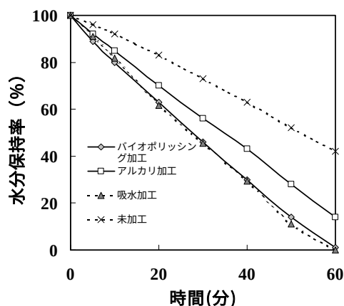
図5 各種加工処理を施した PET 布の速乾性
