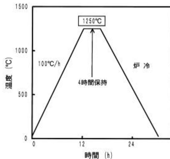
図2 焼結プロセス
