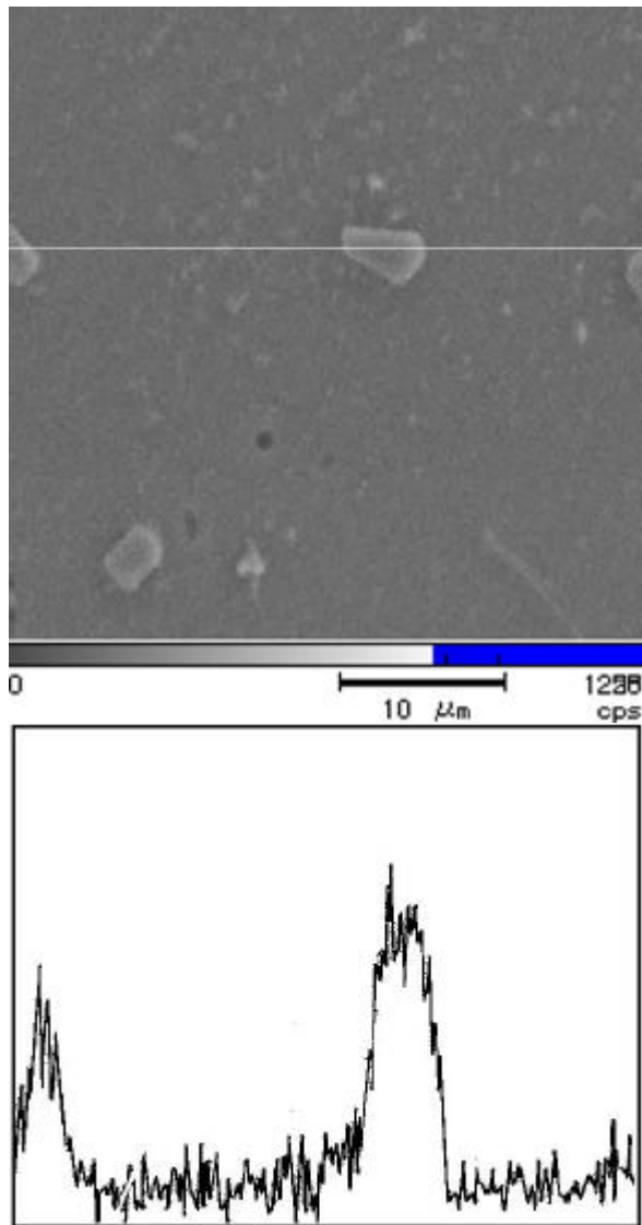
図5 EDSによるSEMとPの線分析
