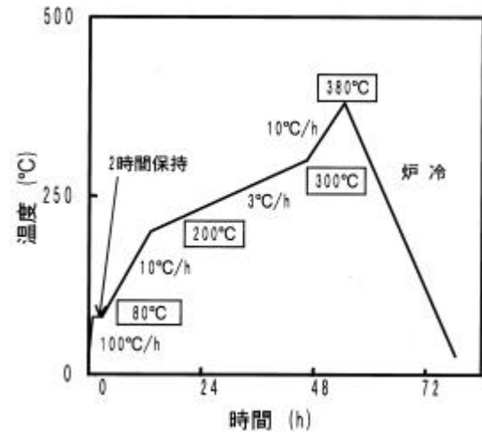
図1 脱脂プロセス
