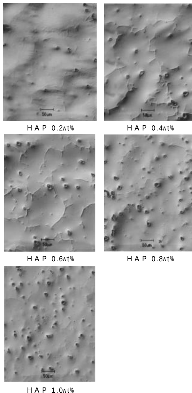
写真3 Ti-HAP 複合材料の光学顕微鏡像 (ノマルスキー微分干渉観察)
