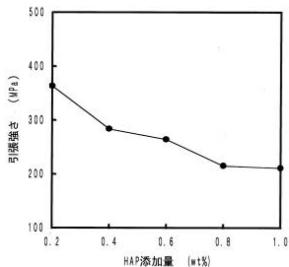
図3 引張り強さとHAP添加量の関係
