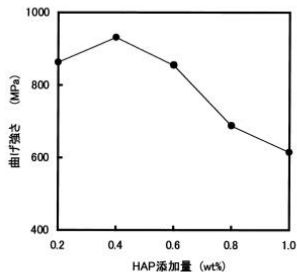
図4 曲げ強さとHAP添加量との関係
