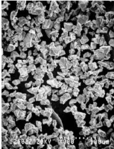
写真1 純チタン粉末の形状
