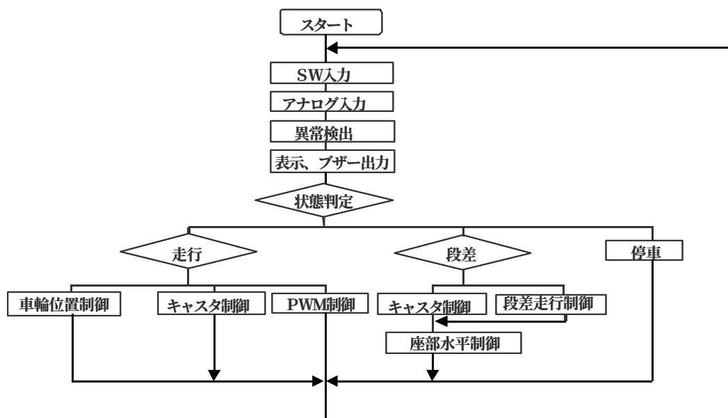
図2 処理の流れ
