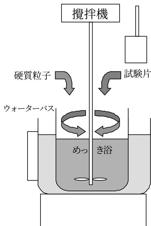
図1 無電解複合めっき装置
