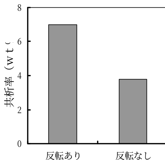
図2 撹拌条件と共析率
