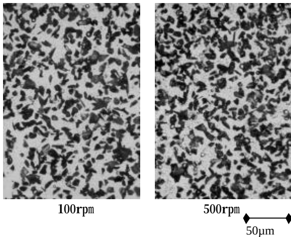
図2 攪拌速度と複合めっきの表面状態
