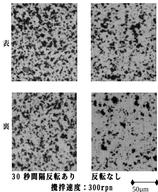
写真1 撹拌方向の有無による複合めっき粒子の分散状態
