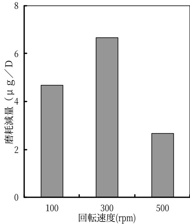
図4 攪拌速度が耐摩耗性に及ぼす影響
