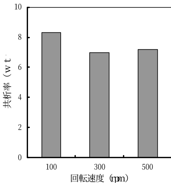
図3 攪拌速度と共析率
