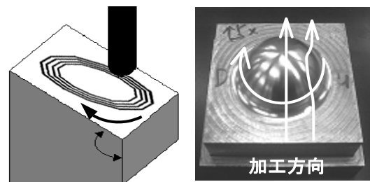
図1 加工姿勢の試験方法
