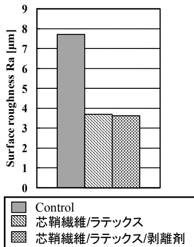
図6 振動試験による表面粗さ
