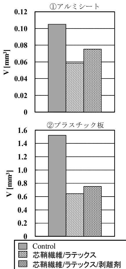
図10 実輸送試験での傷の総量
