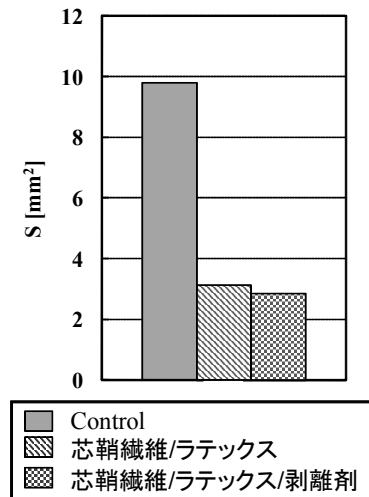
図 5 振動試験による傷の面積
