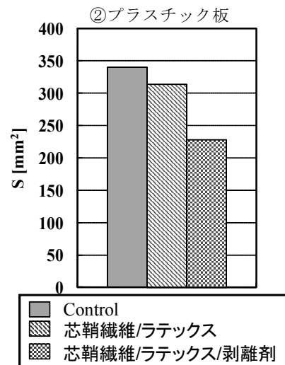
図8 実輸送試験での傷の面積
