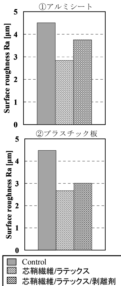
図9 実輸送試験での表面粗さ
