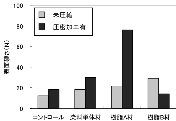
図 7 圧密加工の有無による表面硬さ
