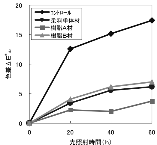
図6 染料単体および樹脂混合含浸試料の耐光性試験による色差変化
