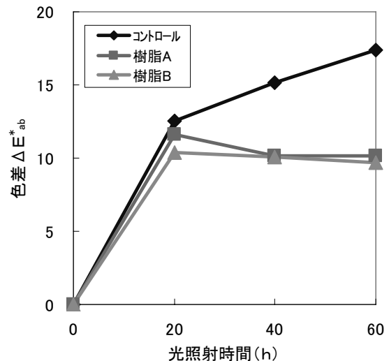
図5 樹脂単体での耐光性試験による色差変化
