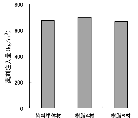
図 2 染料単体および樹脂混合溶液含浸時の薬剤注入量
