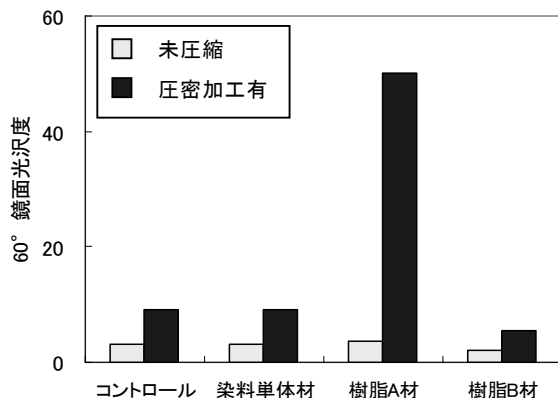
図 8 圧密加工の有無による鏡面光沢度
