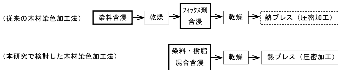
図 1 木材染色加工工程の比較
