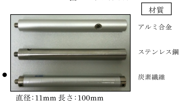
図3 スタイラスエクステンション (EX)
