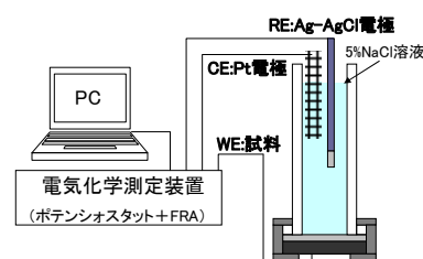
図 1 実験装置の模式図
