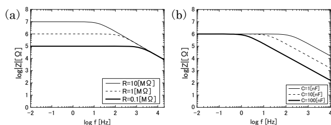
図3 R-C 並列回路のインピーダンススペクトル
