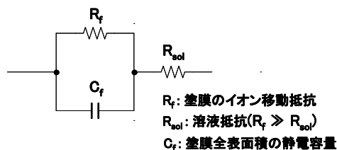
図2 塗膜の等価回路
