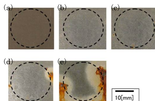
図4 塩水噴霧試験時間経過後の試料表面写真
