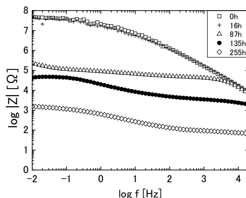
図5 インピーダンススペクトル測定結果
