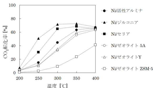
図 6 触媒の CO 2 転化率
