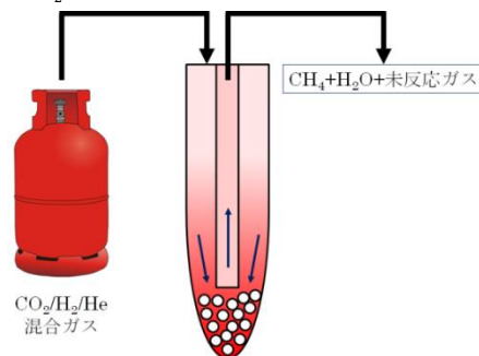
図 1 CO 2 メタン化反応活性評価方法
