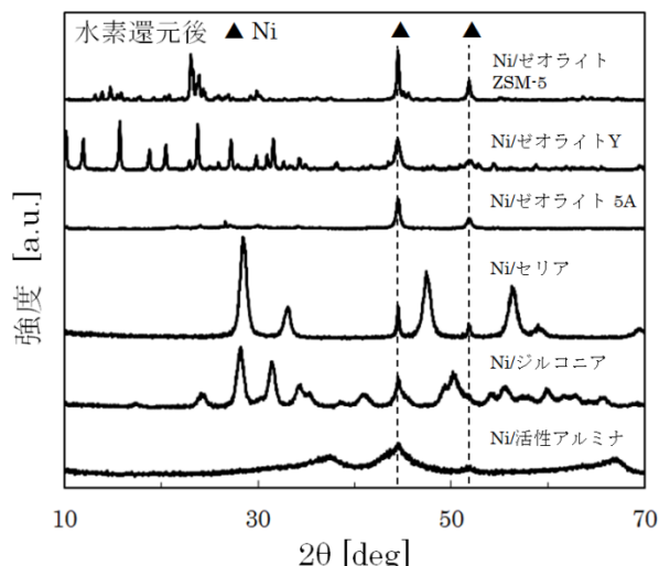
図 3 触媒の XRD 測定結果(水素還元後)
