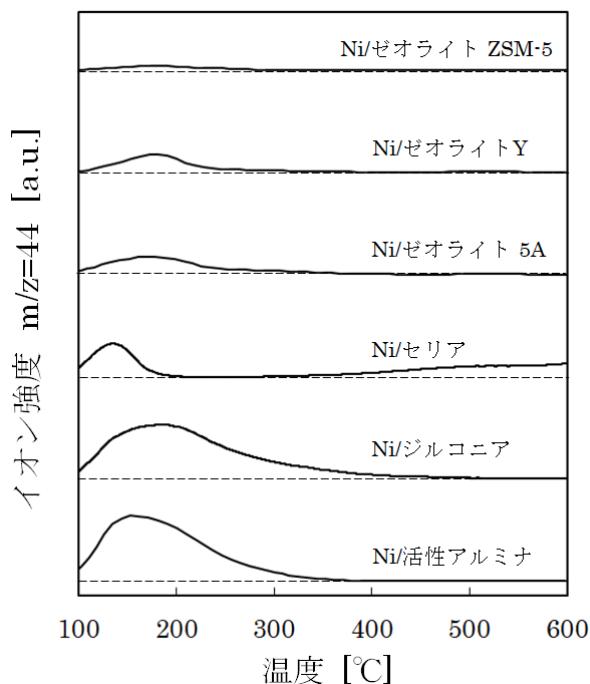
図 8 触媒の CO 2 -TPD 測定
