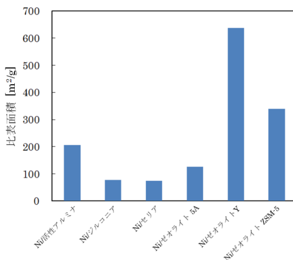
図 4 水素還元後触媒の BET 比表面積
