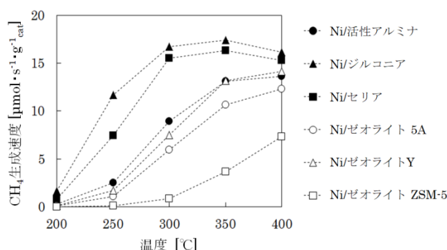
図 7 触媒量あたりの CH 4 生成速度
