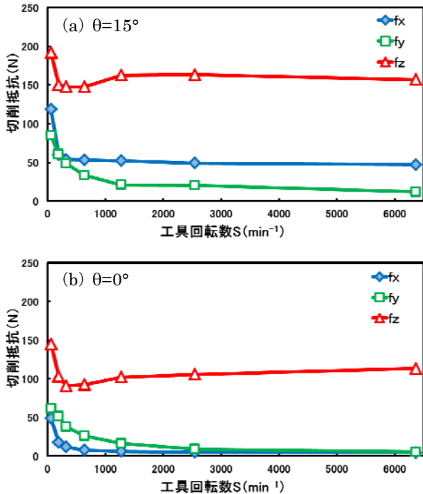
図2 工具回転数と切削抵抗の関係
