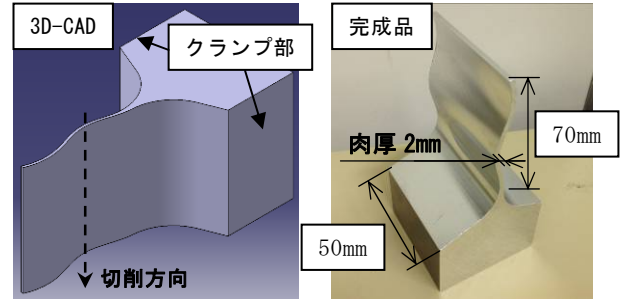
図3 薄肉波形状の加工（肉厚2mm）
