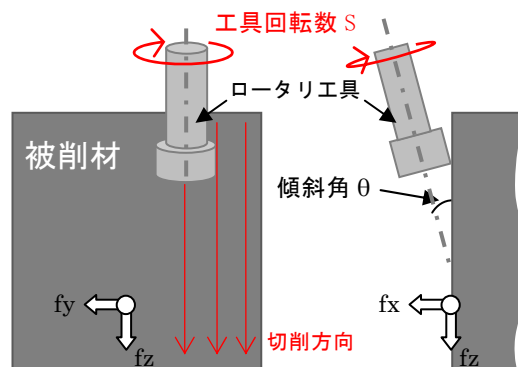
図 1 立ち壁（平面）加工試験の概要
