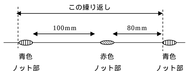
図2 意匠系の模式図
