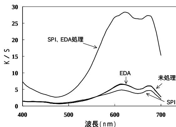
図 1 KayastainQ で染色した各種前処理綿布の K / S 曲線
