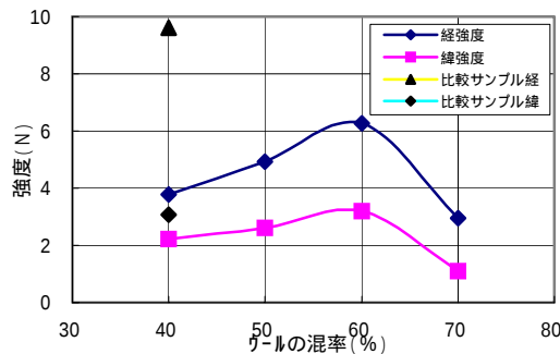
図9 ウールの混率と強度との関係
