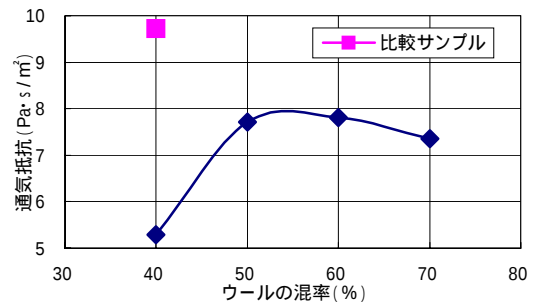
図12 ウールの混率と通気抵抗との関係
