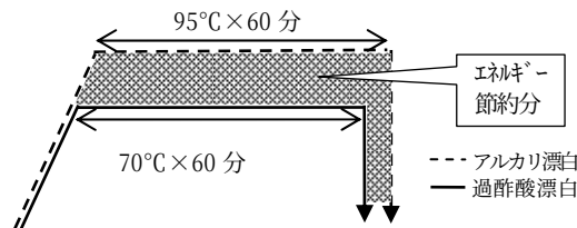
図4 エネルギー使用量の比較
