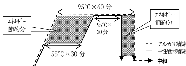
図1 エネルギー使用量の比較
