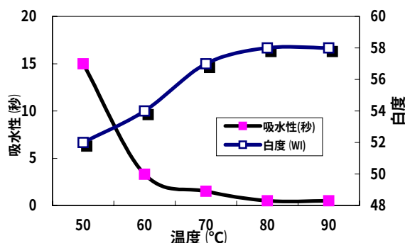
図3 過酢酸の温度の影響
