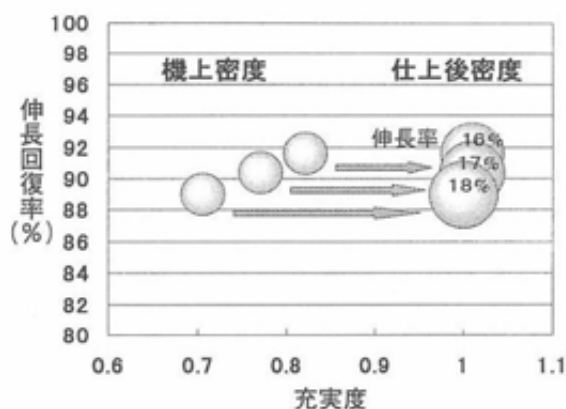
図11 充実度と伸長特性
