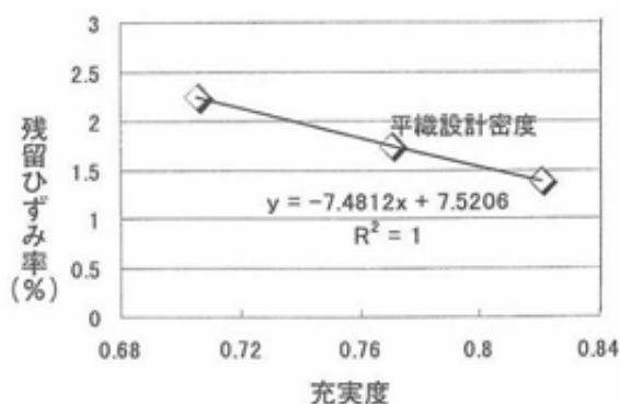
図10 充実度（機上）と残留ひずみ率
