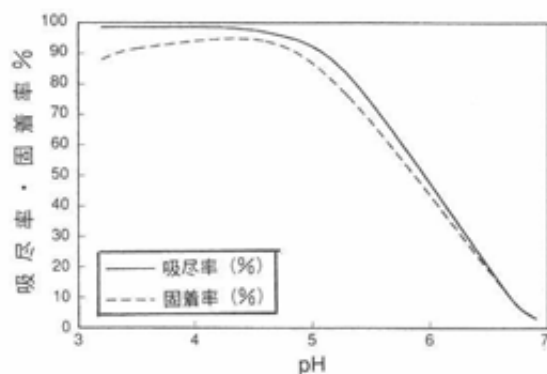
図4 反応染料の吸尽・固着率に及ぼすpHの効果 Sumifix Supra Brill. Red 3BF 2%
