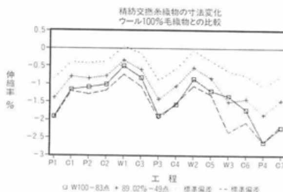
図2 F巻精紡交捻糸織物の寸法変化
