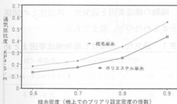
図2 緯糸密度と通気抵抗度
