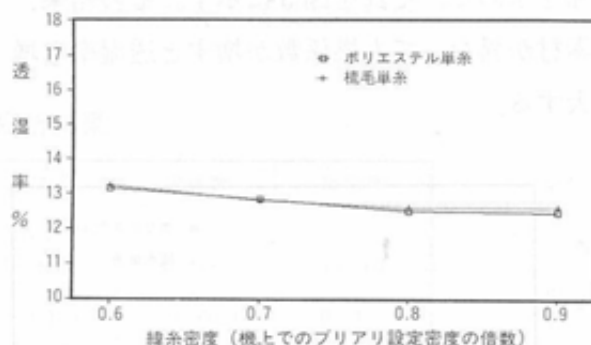
図3 緯糸密度と透湿率
