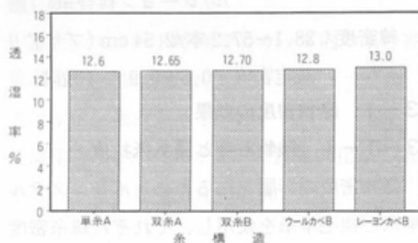
図7 糸構造と透湿率
