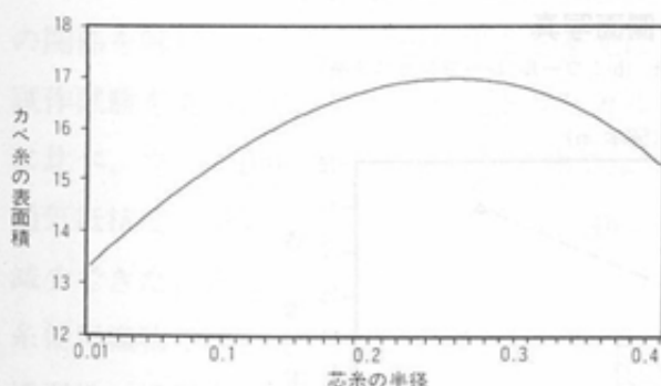
図9 芯糸の半径とカベ糸の表面積 (芯糸と撚糸の断面積の和が一定)
