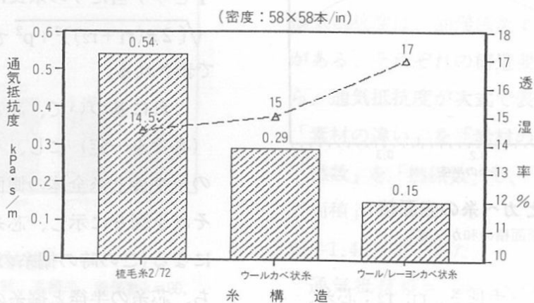
図11 カベ状糸の評価試験結果
