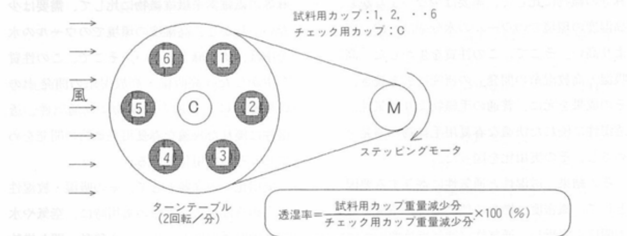
図1 ウォータ法による透湿性測定概念図 (JIS L 1099 A-2法)
