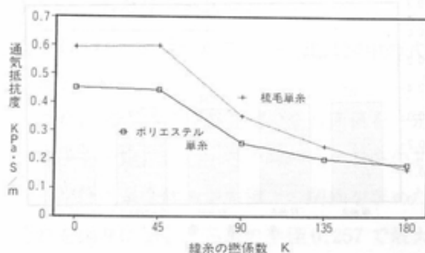
図4 撚係数と通気抵抗度
