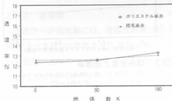
図5 撚係数と透湿率
