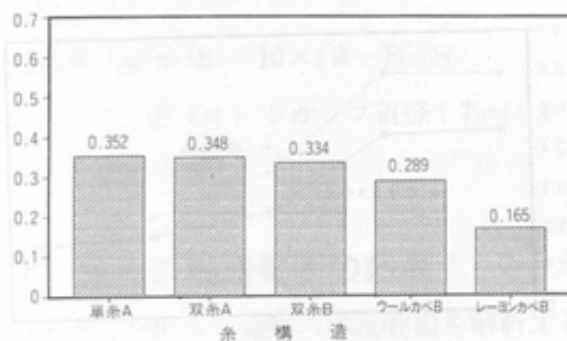
図6 糸構造と通気抵抗度
