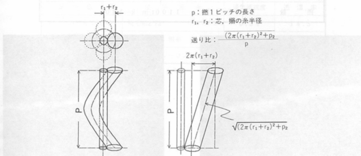
図8 カベ状糸の芯、撚の送り比モデル
