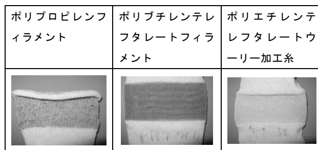
図7 フィラメント系カバリング糸の編成結果
