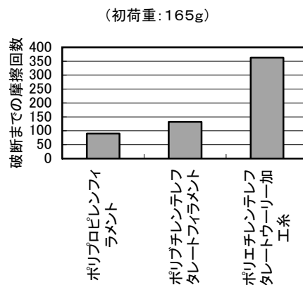
図6 フィラメントカバリング糸の抱合力
