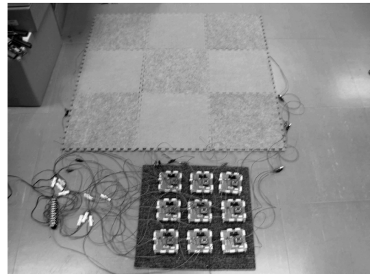
図 11 完成したセンサタイルカーペット
