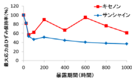
図 2 最大応力点ひずみ保持率推移
