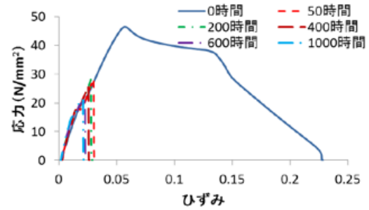
図 4 サンシャインカーボンアーク灯式促進暴露試験後の応力-ひずみ曲線の推移
