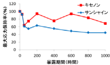
図 1 最大応力保持率推移
