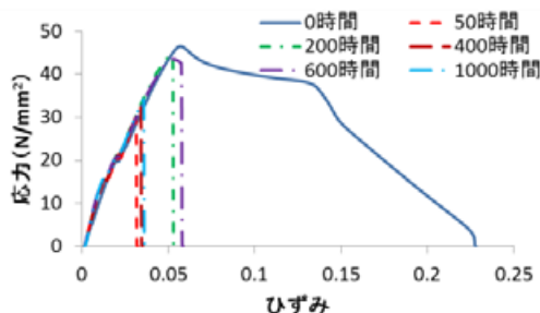
図 3 キセノンアークランプ式促進暴露試験後の応力-ひずみ曲線の推移
