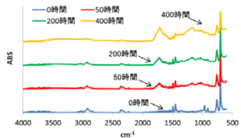
図 5 キセノンアークランプ式促進暴露試験後の赤外吸収スペクトルの推移
