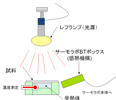
図2 照射蓄熱特性の測定システム
