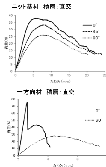
図 8 曲げ試験結果（荷重－たわみ曲線）
