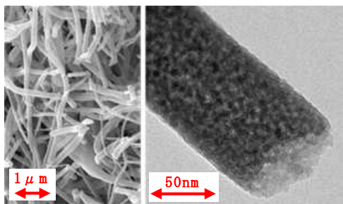
作成した多孔質酸化チタン ナノファイバーの拡大写真
