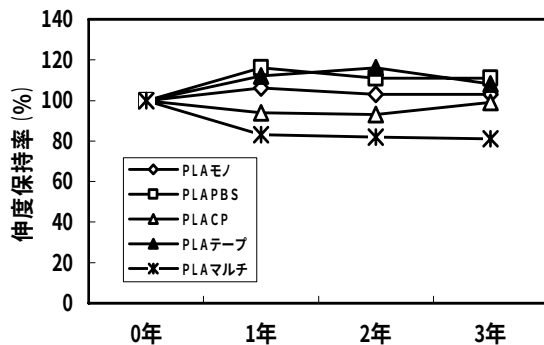
図4 ロープの伸度保持率（岡崎市土中）
