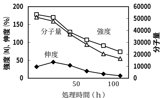
図8 高温・高湿試験による強度、伸度、分子量変化
