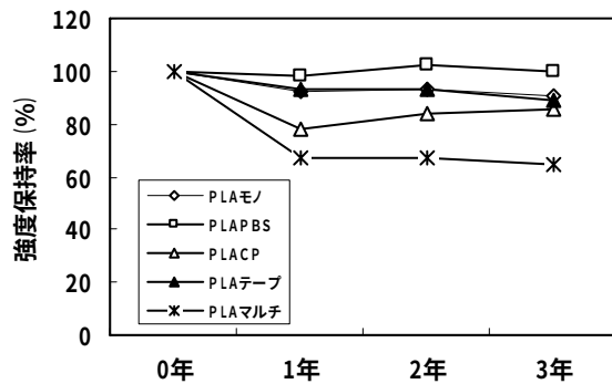
図3 ロープの強度保持率（岡崎市土中）
