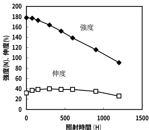
図7 サンシャインウエザーメータによる促進劣化
