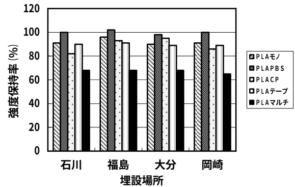
図6 ロープの強度保持率（場所による違い）
