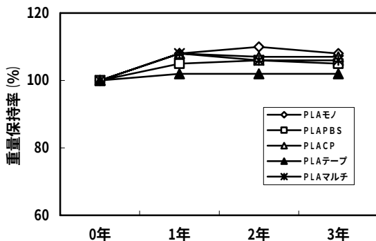
図5 ロープの重量保持率（岡崎市土中）
