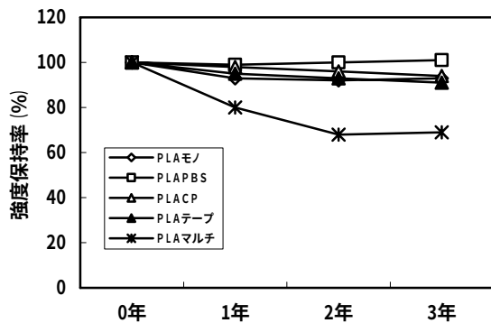
図6 ロープの強度保持率（屋外暴露）
