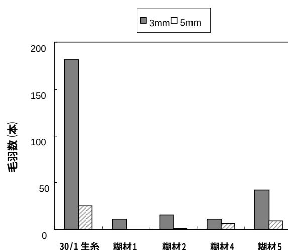
図2 糊付けにおける毛羽数の変化
