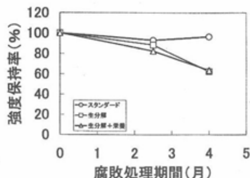
図11 付着海苔腐敗処理による網の強度保持率
