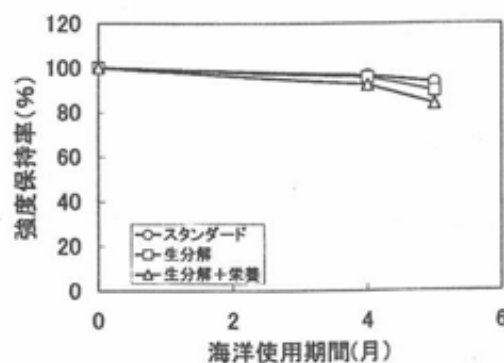
図 10 海洋使用による網の強度保持率
