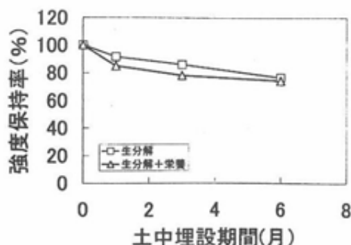
図12 土中埋設によるトワイン強度保持率
