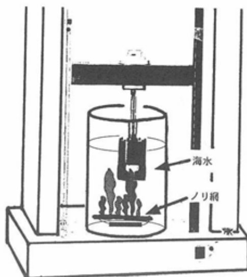
図1 海苔葉体付着強度の測定法
