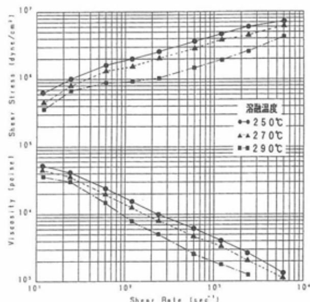
図3 熔融温度と流動特性(カーボン含有量25%)
