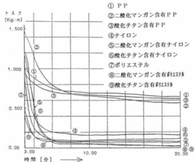
図1 樹脂の流動特性
