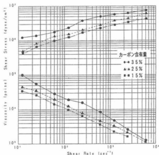
図2 カーボン含有量と流動特性(熔融温度270℃)
