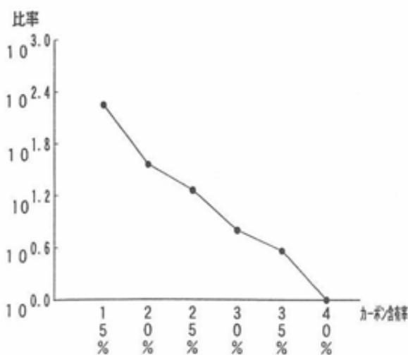
図5 カーボン40%に対する電気抵抗値の比(未延伸糸)
