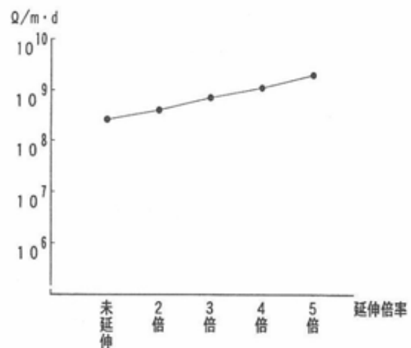
図6 延伸倍率と電気抵抗(カーボン15%)
