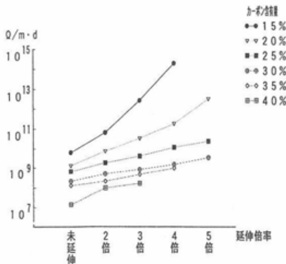
図4 カーボン含有率、延伸倍率と電気抵抗
