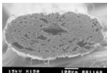
図2 発泡 LL/PLA 繊維 断面
