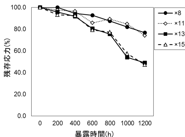
図2 延伸倍率の違いにおける暴露時間に対する残存応力(荷重負荷有)
