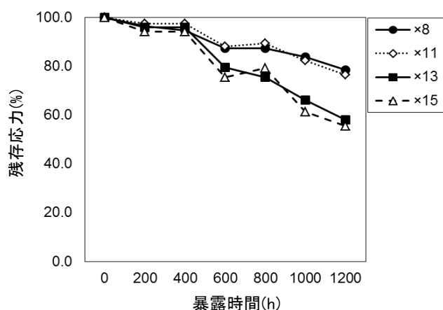
図1 延伸倍率の違いにおける暴露時間に対する残存応力(荷重負荷無)
