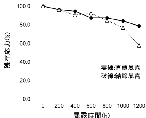
図3 延伸倍率8倍における直線暴露と結節暴露の暴露時間に対する残存応力
