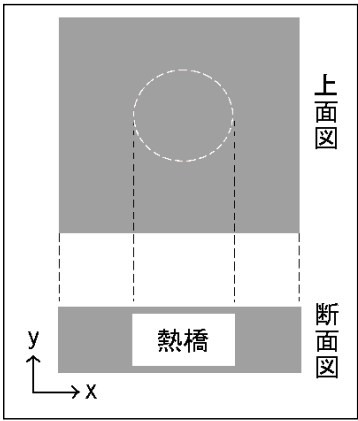
図2 熱橋形成タイル模式図
