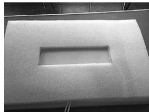
図5 加熱試験 ウレタンフォームでタイル側面及びヒーター下面を断熱した状態
