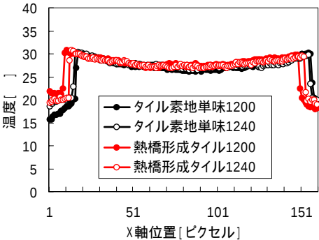
図11 タイル表面の温度分布
