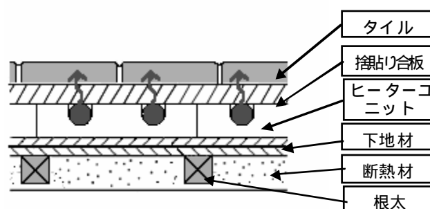
図1 床暖房の床構造（根太上設置方式）
