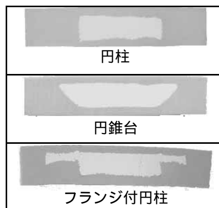
写真 熱橋形成タイルの切断面
