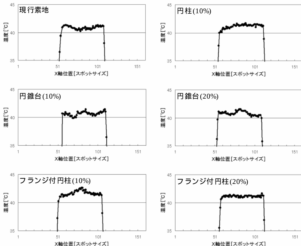
図6 タイル表面中央を横断する線上の温度分布（1240 焼成体）
