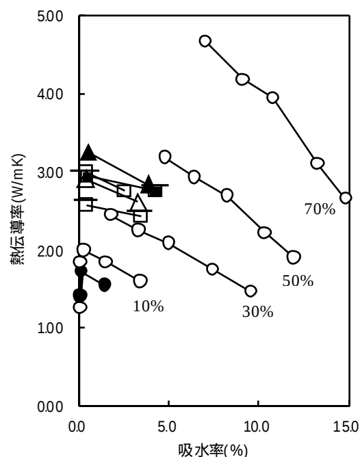
図3 熱橋形成タイルの熱伝導率と吸水率
