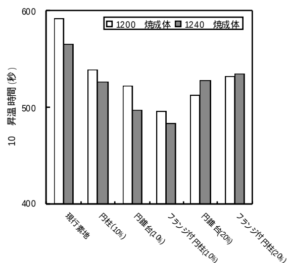
図4 熱橋形成タイルの昇温特性
