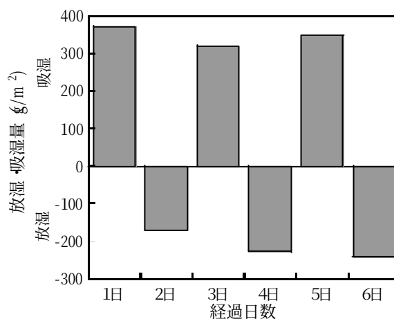
図10 試作品の調湿特性 50RH%～90RH%)
