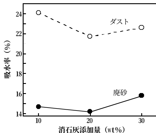
図6 ベントナイト系固化体の吸水率 (熱処理温度：1100°C)
