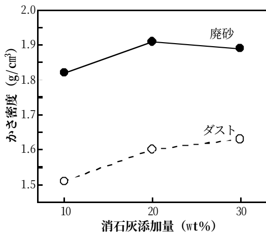
図2 ベントナイト系成形体のかさ密度 (熱処理温度：1100°C)
