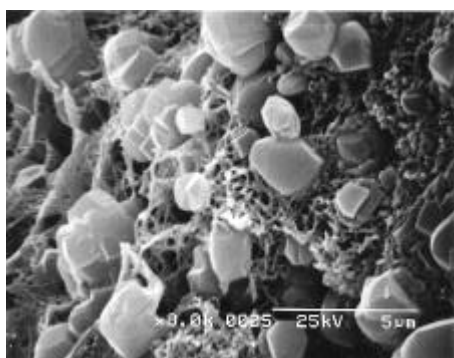
写真 固化体の破断面の SEM 写真 (水ガラス系廃砂 80wt% 消石灰 20wt%)
