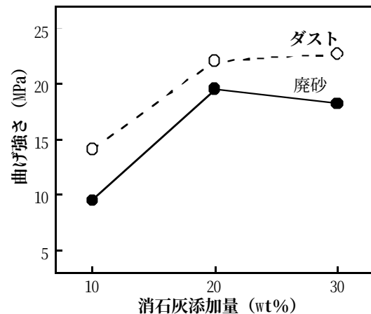
図4 ベントナイト系固化体の曲げ強さ (熱処理温度：1100°C)
