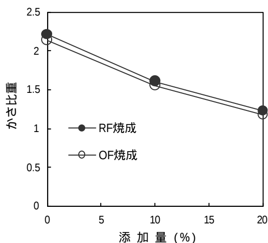
図5 活性炭(細粒)添加量とかさ比重
