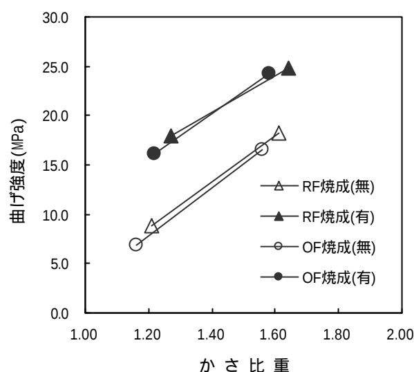
図7 曲げ強度に対する表面熔化化粧土の効果
