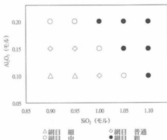
図3 オートクレープ処理後の貫入発生状況 (1140°C)
