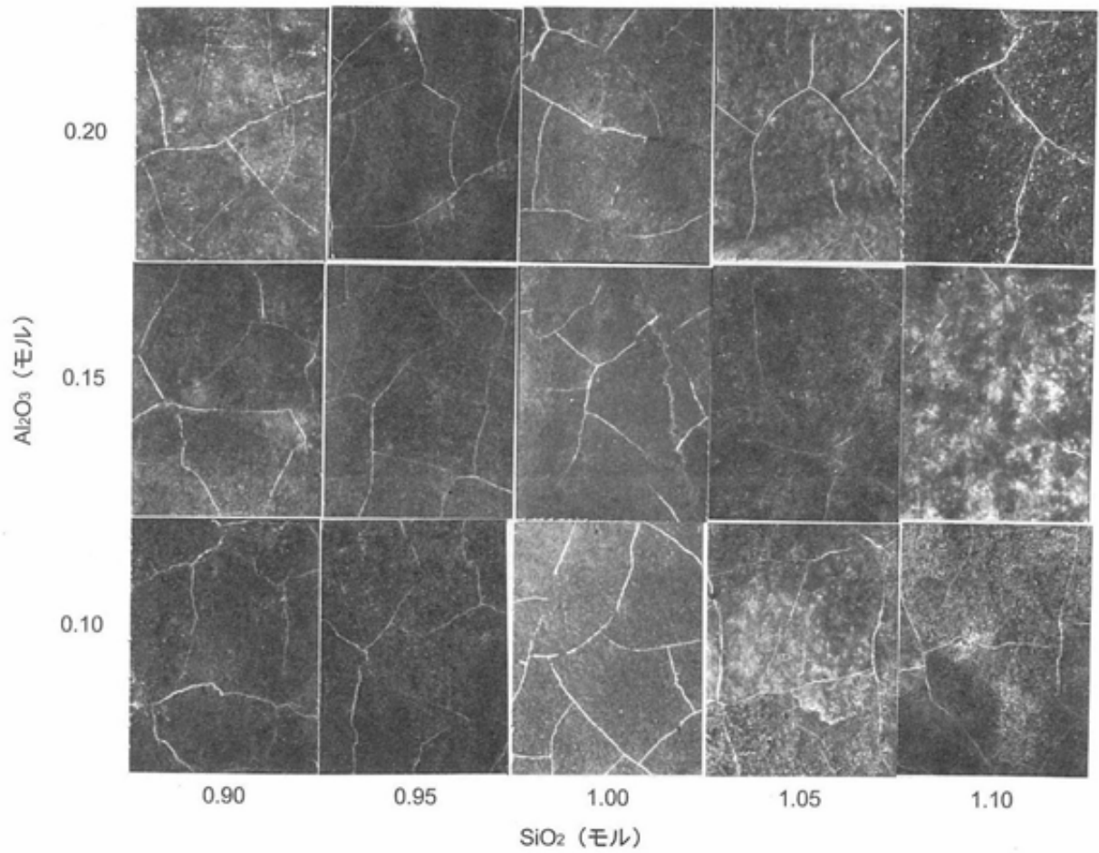
写真1 オートクレープ処理後貫入発生状況 (1140°C)
