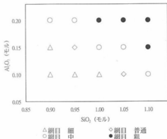
図2 オートクレープ処理後の貫入発生状況 (1120°C)
