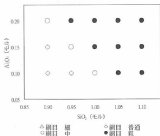
図4 オートクレープ処理後の貫入発生状況 (1160°C)
