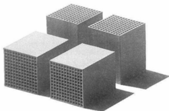
写真 スラグハニカム低温焼成体 (左：900℃, 右：1000℃)
